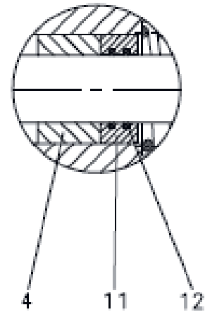
EINZELHEIT X
