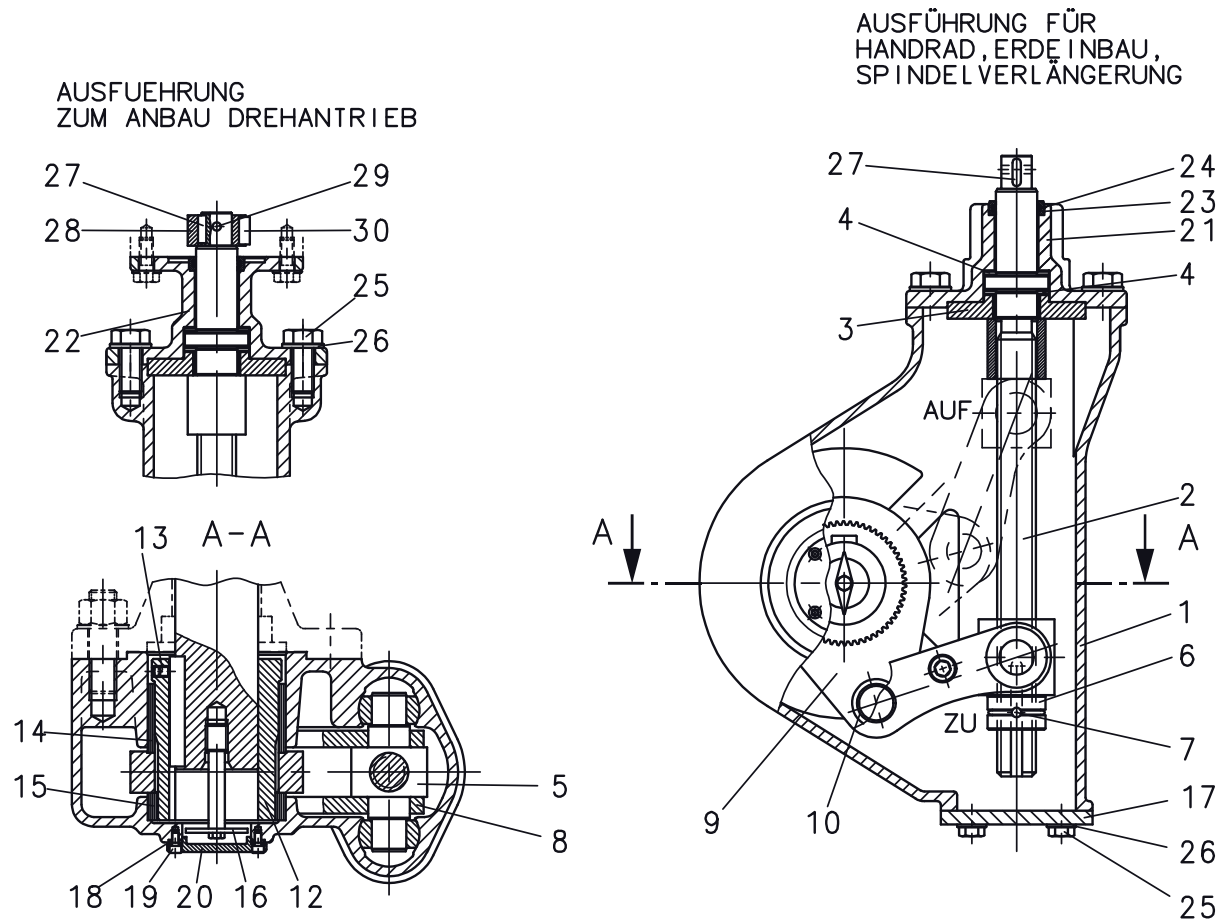
Abbildung 8: Schnittbild SKG-Schubkurbelgetriebe
